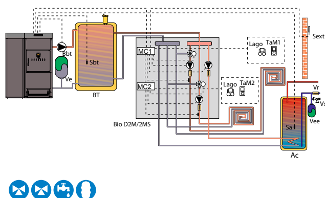
MODUL BIO D2M/2MS + BT
