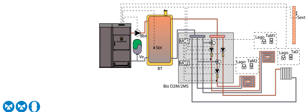
MODUL BIO D2M/2MS + BT
