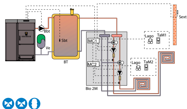
MODUL BIO 2M + BT
